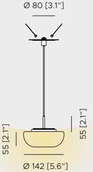
WITHOUT CANOPY / SENZA ROSONE
