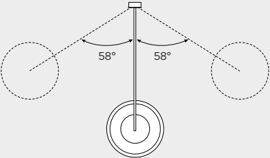
ARM ROTATION / ROTAZIONE DEL BRACCIO
