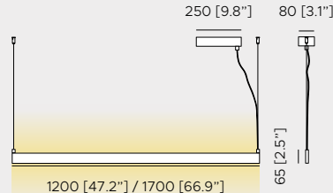
WITHOUT SHADE / SENZA PARALUME
