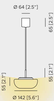
WITH CANOPY / CON ROSONE
