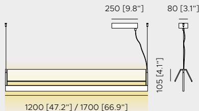
WITH SHADE / CON PARALUME
