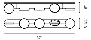
37" VL72237
