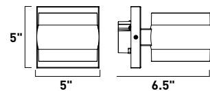
E30171-10BK Wall Mount
