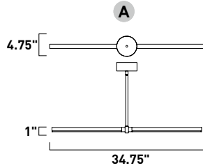
E21355-BK, -GLD, -PC Pendant
