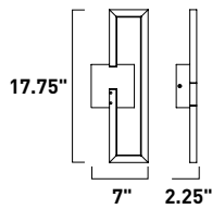
E21260-BK, -GLD ADA Compliant Wall Mount
