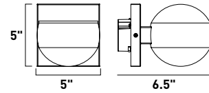
E30165-10BK Wall Mount
