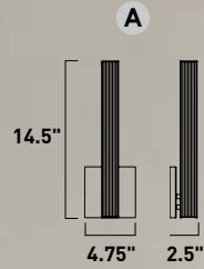
E11060-144BK, -144NAB Wall Mount
