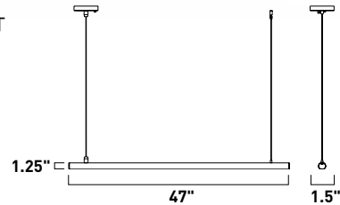
E26004-90BK, -90SA, -90WT Pendant
