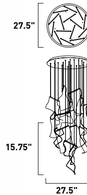
E24877-133BGM, -133FG, -133PC Pendant
